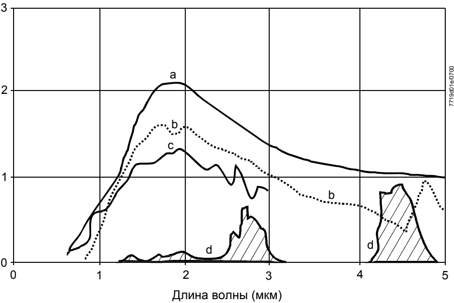
Спектральная эмиссия излучения светящегося и несветящегося пламени при 1,500 К (выписка из VDI Отчета no. 423, 1981).
