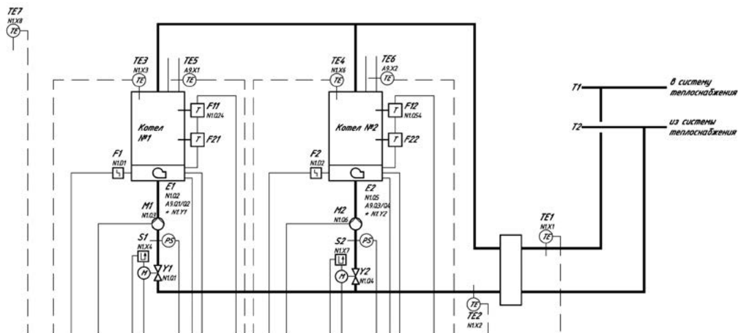
Каскад с двумя котлами на контроллере RMK770-1
