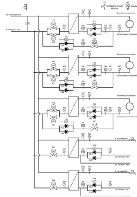
Принципиальная схема теплового пункта для управления 3 контурами отопления и 2 контурами ГВС
