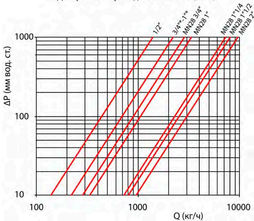
Диаграмма перепада по нефти (вязкость ≤3°E)
