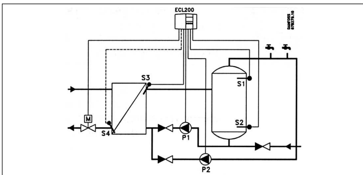
Рис. 7. Схема применения – 2.
