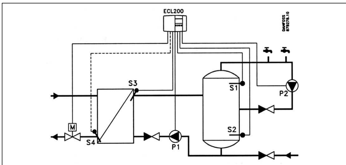
Рис. 6. Схема применения – 1.
