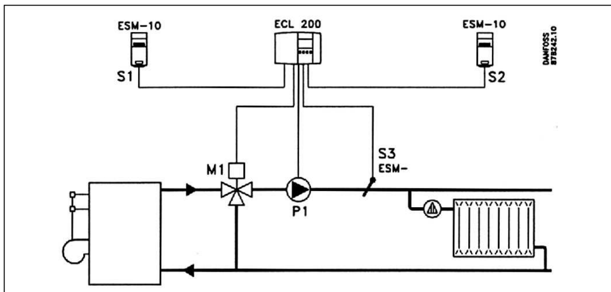
Рис. 11. Схема применения –3.
