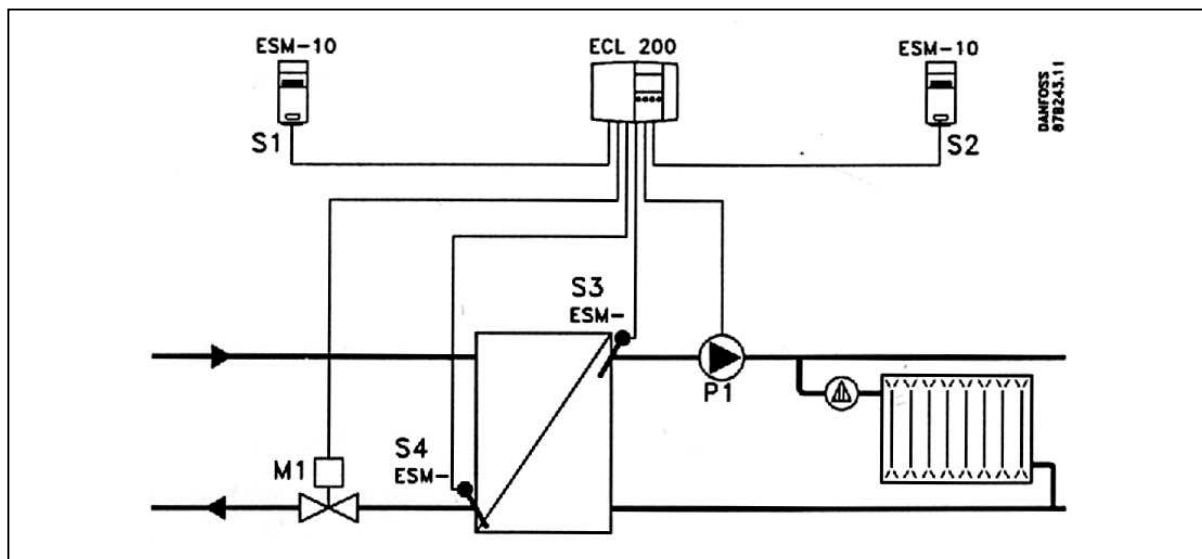
Рис. 9. Схема применения –1.
