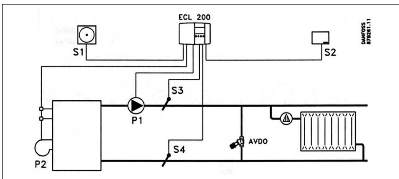
Рис. 8. Схема применения.
