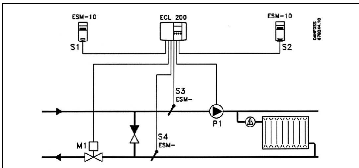
Рис. 10. Схема применения –2.
